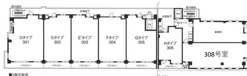
3階平面図
