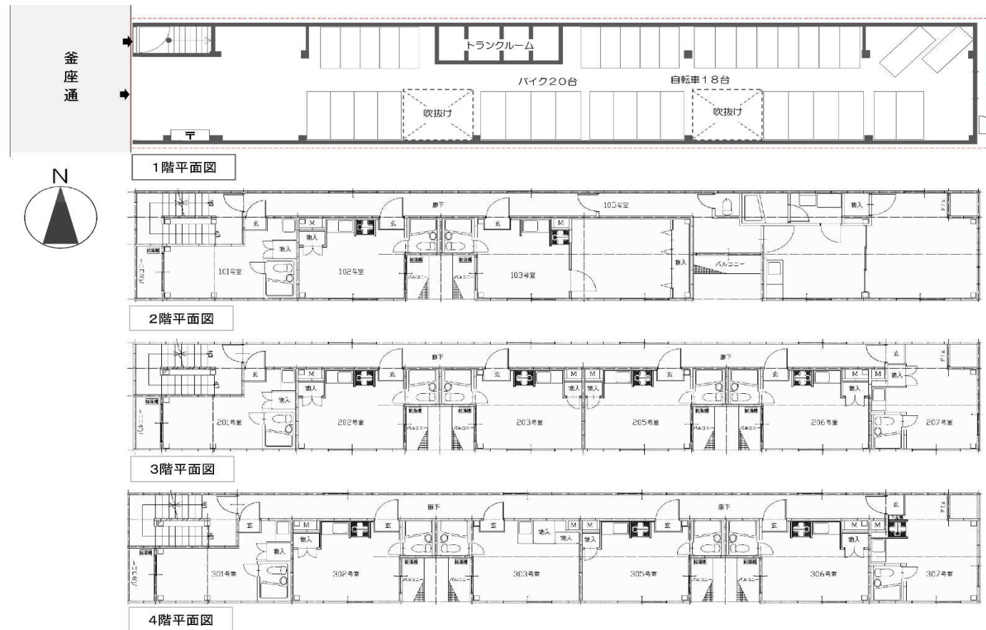
各階平面図
