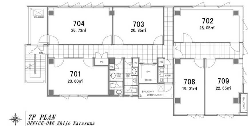
7階平面図
