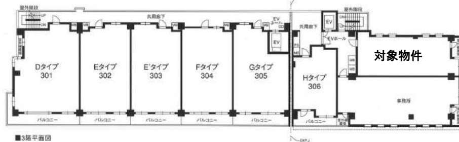
3階平面図
